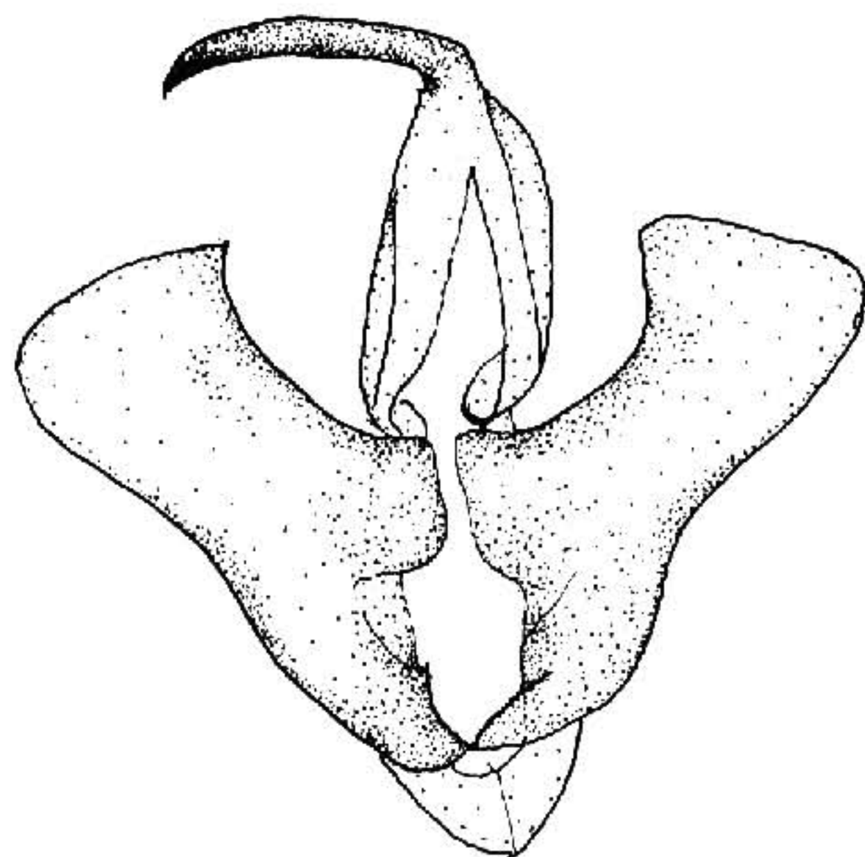
图 680 闪疔夜蛾 Adrapsa simplex (Butler) ♂ 外生殖器
