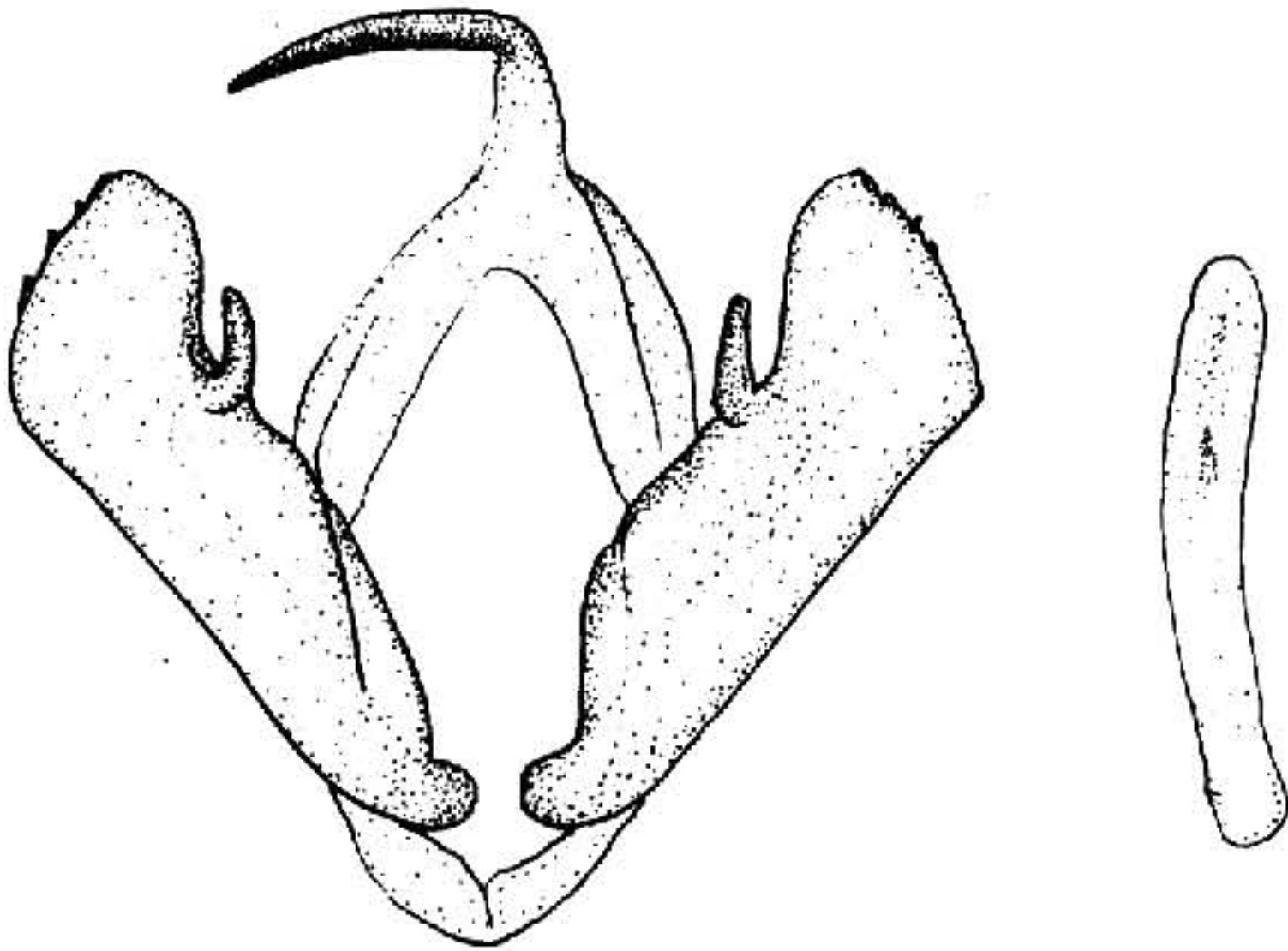
图 679 点疖夜蛾 Adrapsa notigera (Butler) ♂ 外生殖器
